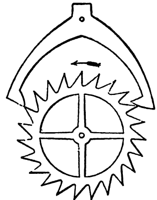
FIG. 4.—Anchor Escapement.
