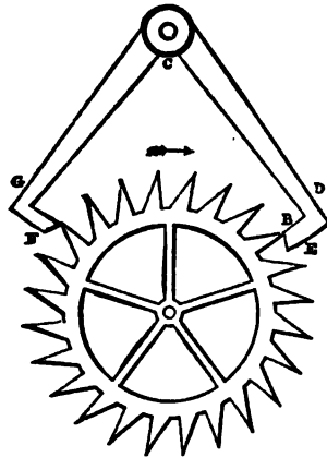
FIG. 5.—Dead Escapement.
