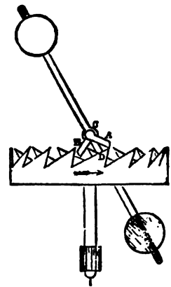
FIG. 3.—Recoil Escapement.
