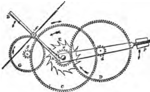
FIG. 20.—Gravity Train Remontoire.
