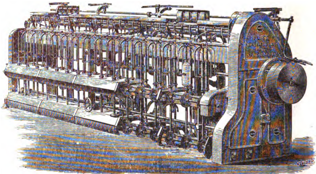
FIG. 9.—Slubbing Frame.
