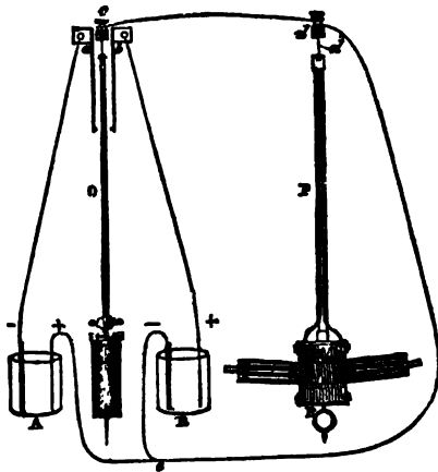
FIG. 16.—Bain's Pendulum.
